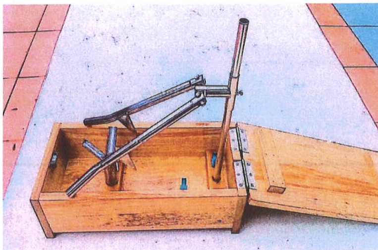
ภาพที่ 1 อุปกรณ์สำหรับปอกเปลือกทุเรียนแบบ Knock Down (กึ่งกลาง ขนาด 16 pt.) (ตัวหนา)
