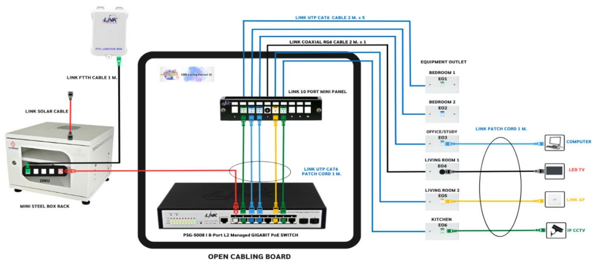
รูปที่ 6 การเชื่อมต่อและตำแหน่งการติดตั้งอุปกรณ์ทั้งระบบ
